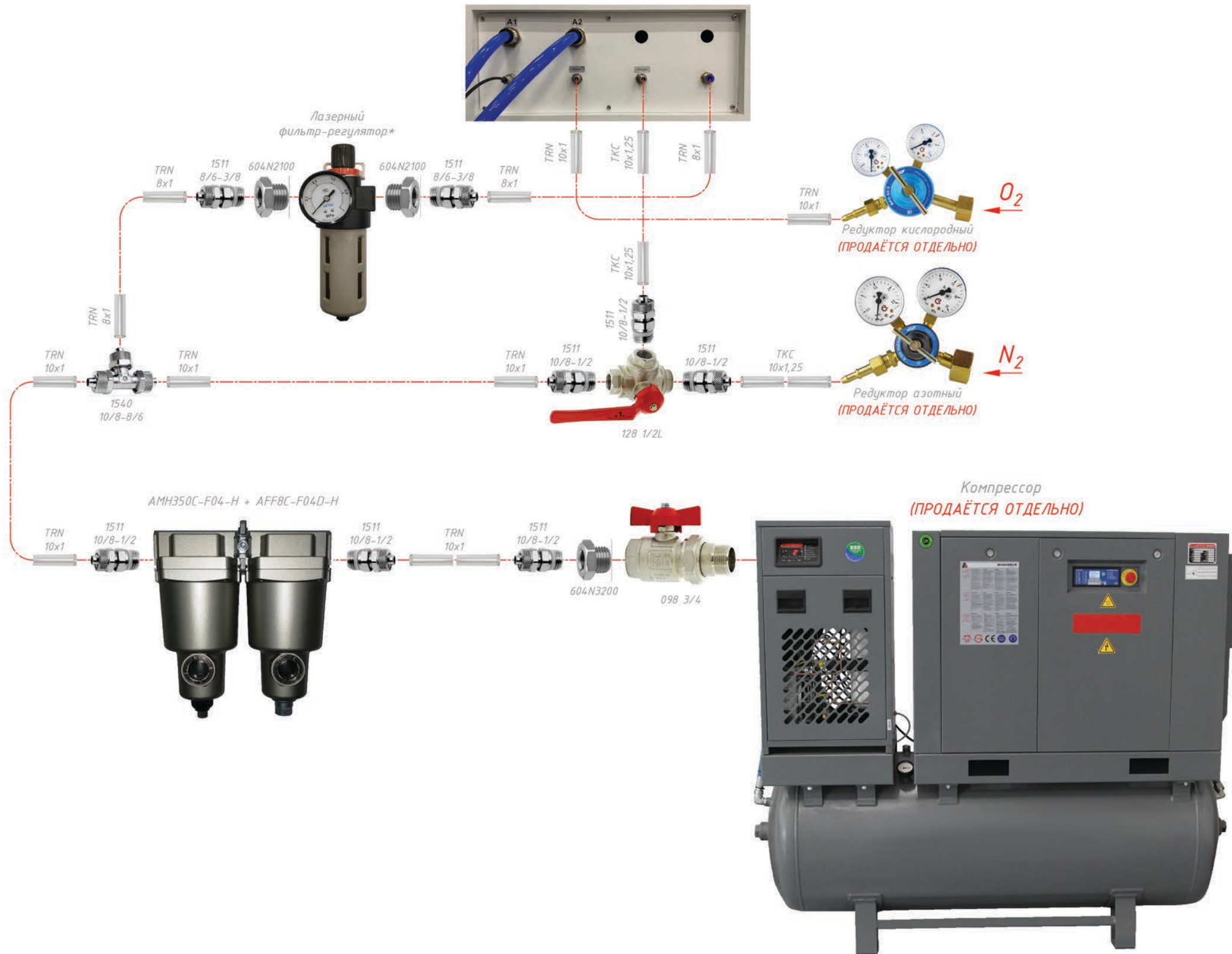
Задняя панель лазерной установки
